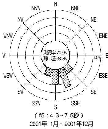
付図 - B.2.44 高知 波高・波向別出現頻度図 ( f2 , f3 , f4 , f5 , 全周期帯 )
