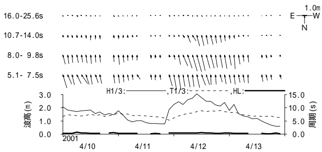
付図 - B.1.20 那覇 周期帯別波浪特性の経時変化(高波期間中)
