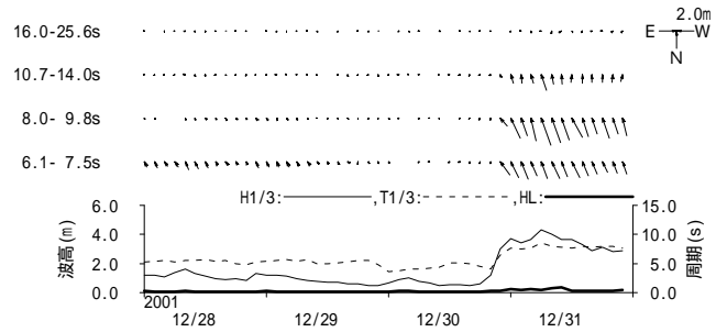
付図 - B.1.22 紋別(南) 周期帯別波浪特性の経時変化(高波期間中)
