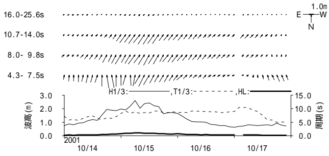
付図 - B.1.21 紋別 周期帯別波浪特性の経時変化(高波期間中)
