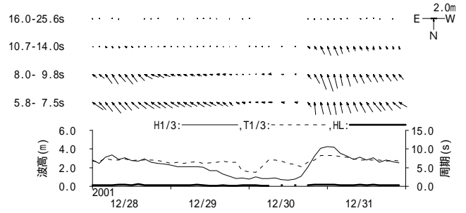
付図 - B.1.1 留萌 周期帯別波浪特性の経時変化(高波期間中)
