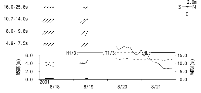
付図 - B.1.47 宮崎 周期帯別波浪特性の経時変化(高波期間中)
