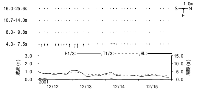
付図 - B.1.46 苅田 周期帯別波浪特性の経時変化(高波期間中)
