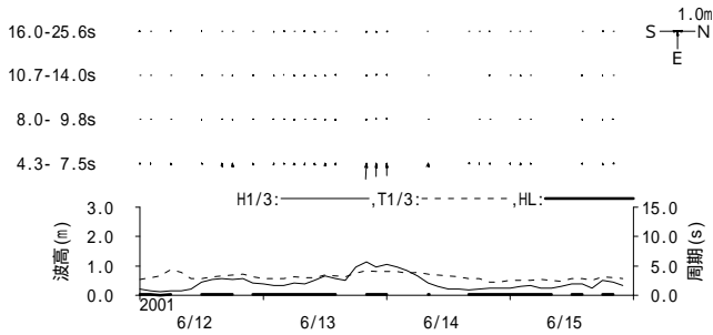
付図 - B.1.46 苅田 周期帯別波浪特性の経時変化(高波期間中)
