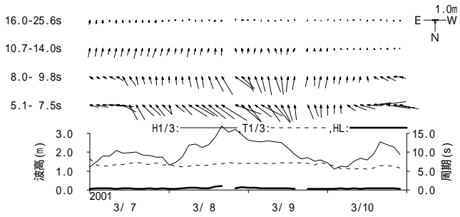
付図 - B.1.17 玄界灘 周期帯別波浪特性の経時変化(高波期間中)
