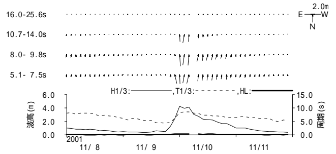
付図 - B.1.17 玄界灘 周期帯別波浪特性の経時変化(高波期間中)
