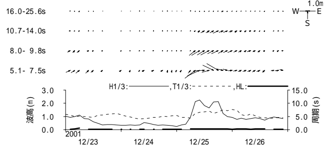
付図 - B.1.18 伊王島 周期帯別波浪特性の経時変化(高波期間中)
