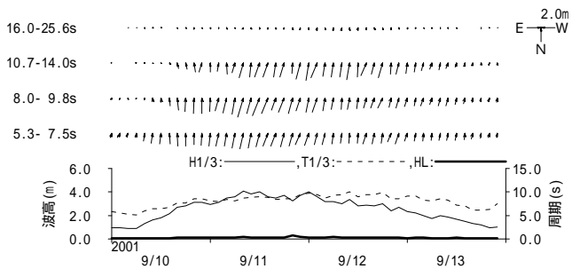
付図 - B.1.11 柴山 周期帯別波浪特性の経時変化(高波期間中)
