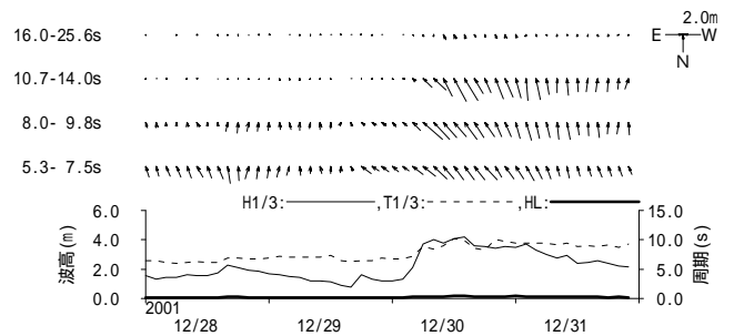
付図 - B.1.11 柴山 周期帯別波浪特性の経時変化(高波期間中)
