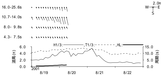
付図 - B.1.44 高知 周期帯別波浪特性の経時変化(高波期間中)
