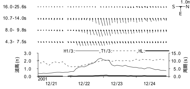
付図 - B.1.30 相馬 周期帯別波浪特性の経時変化(高波期間中)
