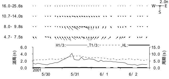
付図 - B.1.36 波浮 周期帯別波浪特性の経時変化(高波期間中)
