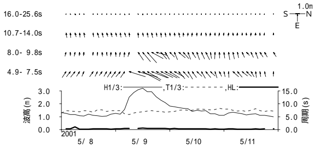
付図 - B.1.32 常陸那珂 周期帯別波浪特性の経時変化(高波期間中)
