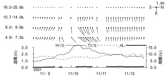
付図 - B.1.32 常陸那珂 周期帯別波浪特性の経時変化(高波期間中)
