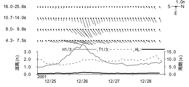
付図 - B.1.33 鹿島 周期帯別波浪特性の経時変化(高波期間中)
