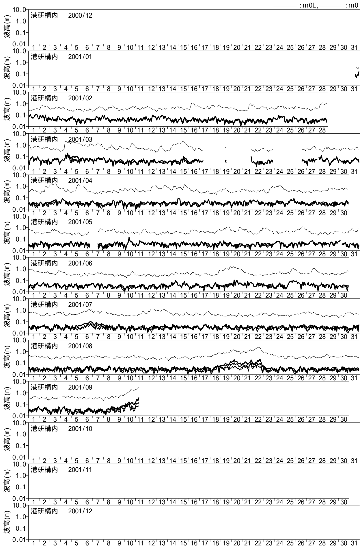
付図 - A.2.35 長周期波高の経時変化図 (港研構内)
