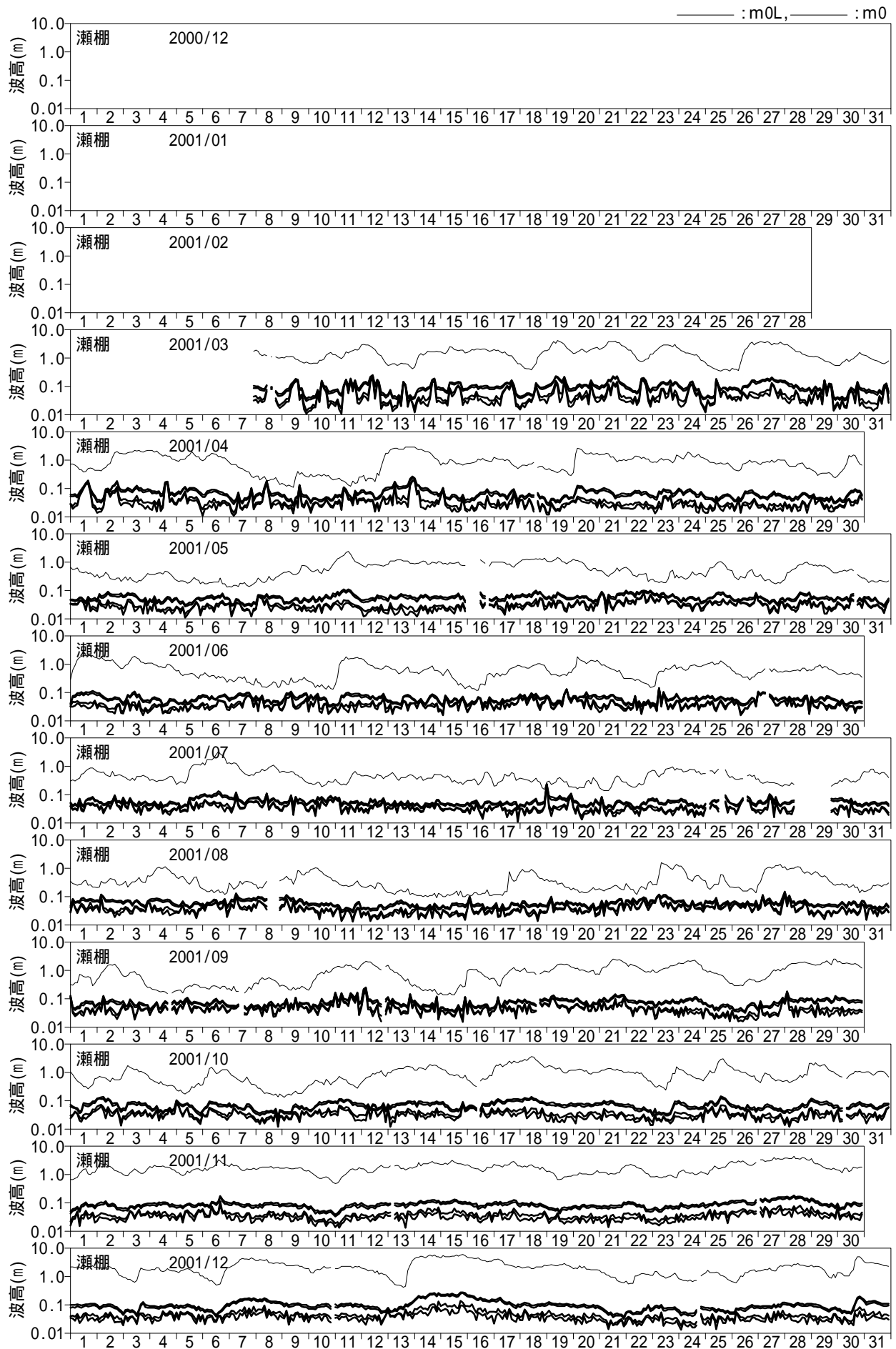
付図 - A.2.2 長周期波高の経時変化図 (瀬棚)
