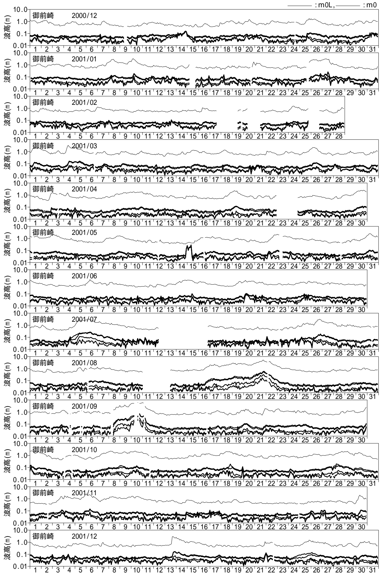
付図 - A.2.39 長周期波高の経時変化図 (御前崎)
