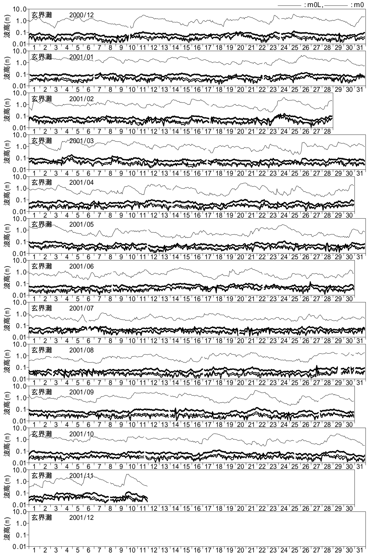
付図 - A.2.17 長周期波高の経時変化図 (玄界灘)
