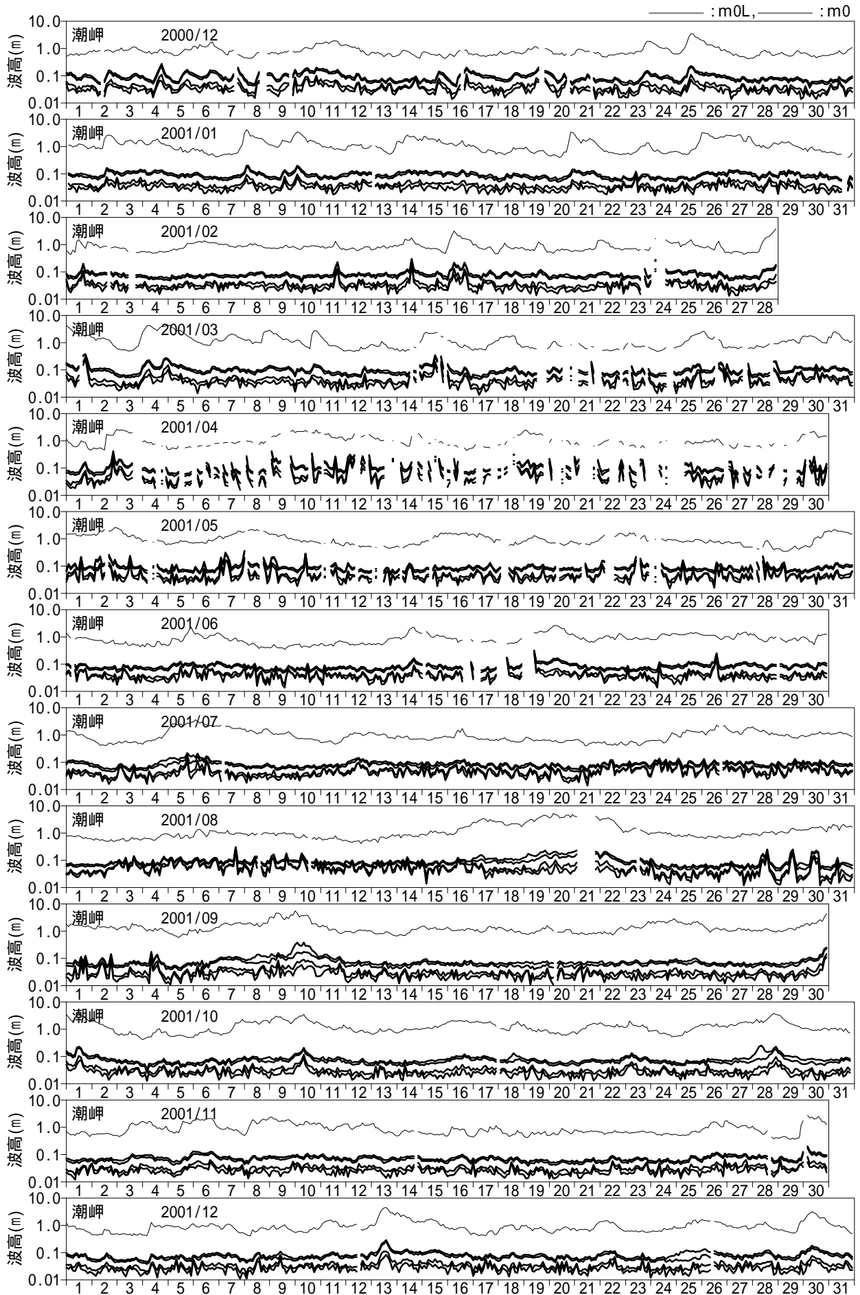
付図 - A.2.40 長周期波高の経時変化図 (潮岬)
