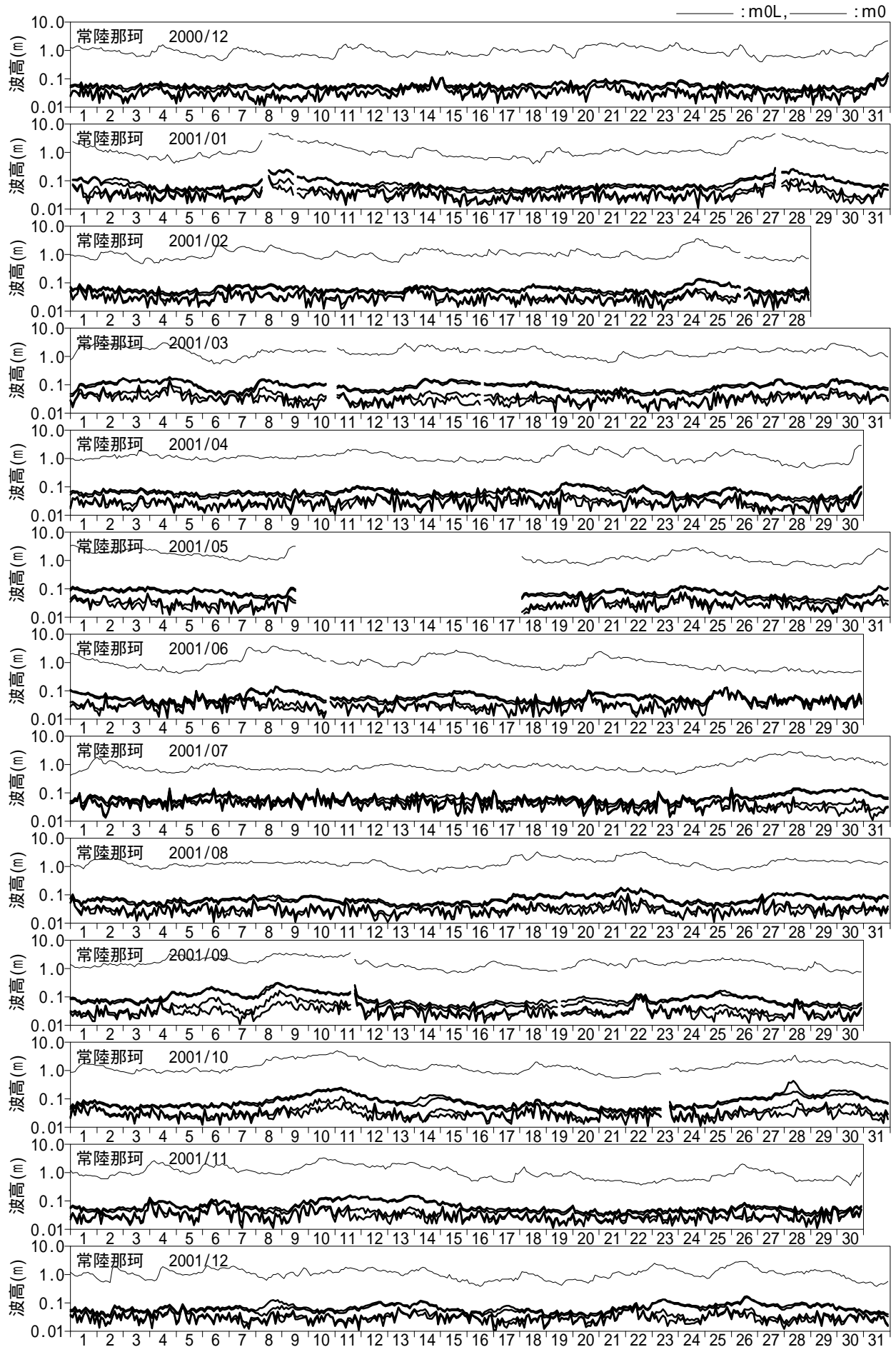
付図 - A.2.32 長周期波高の経時変化図 (常陸那珂)
