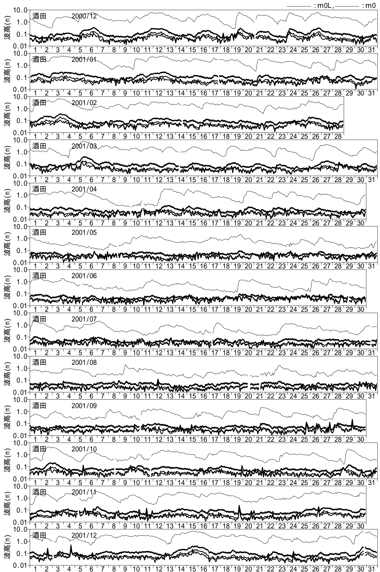
付図 - A.2.5 長周期波高の経時変化図 (酒田)
