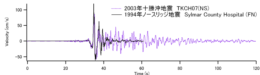
図-1 海溝型巨大地震と内陸地殻内地震によるパルス波の比較例
